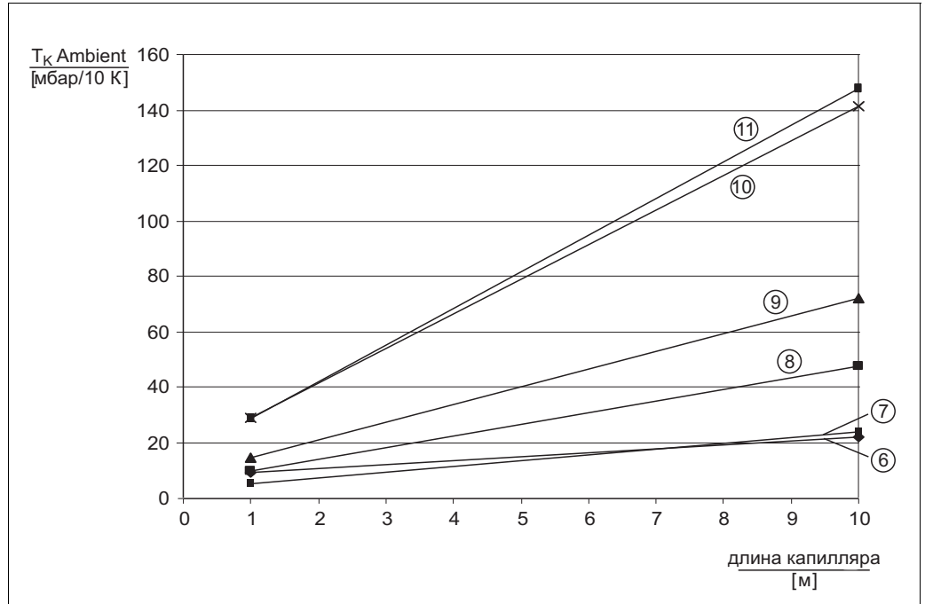
Диаграмма зависимости T_k Ambient от длины капилляра для PMP46
