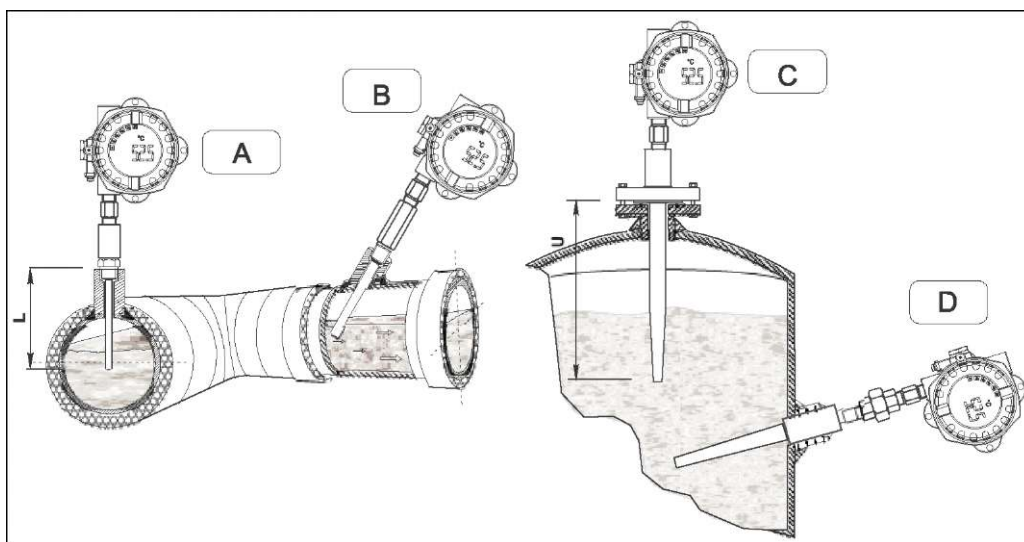
Примеры монтажа
