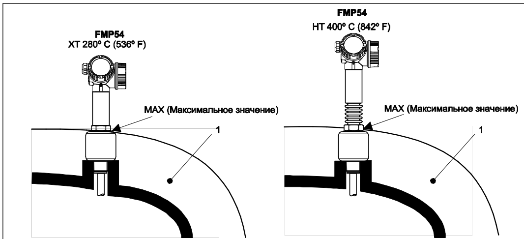
1 Изоляция резервуара
