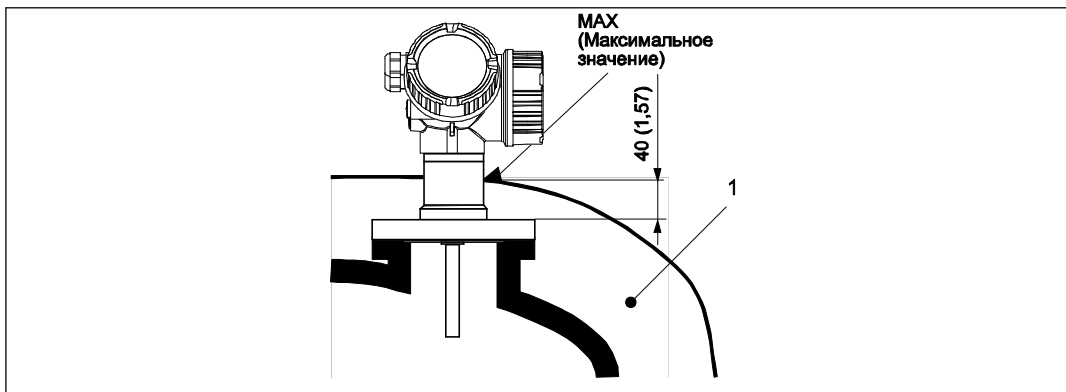
1 Изоляция резервуара
