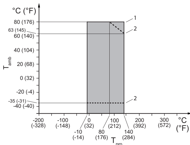
Рис. 18. Допустимая температура рабочей среды и окружающей среды, разнесенное исполнение, для типа присоединения к технологическому процессу HS4 и HS8
