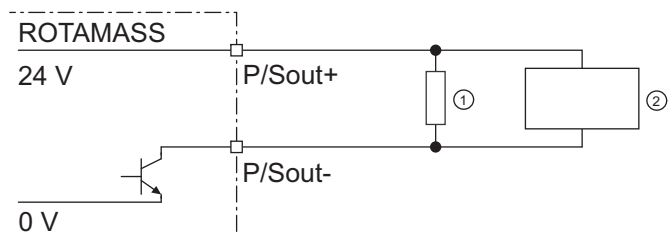
Рис. 26. Соединение активного импульсного выхода P/Sout
