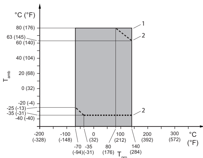
Рис. 17. Допустимая температура рабочей среды и окружающей среды, разнесенное исполнение, для типа присоединения к технологическому процессу HS2
