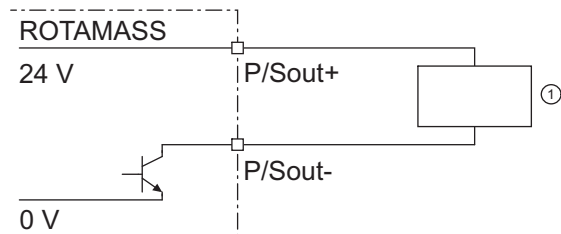
Рис. 31. Соединение активного выхода состояния P/Sout
