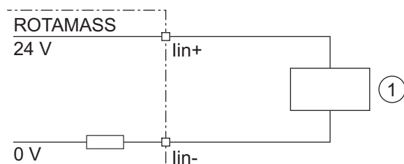
Рис. 36. Подсоединение внешнего устройства с пассивным токовым выходом
