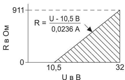
Рис. 24. Максимальное сопротивление нагрузки как функция напряжения внешнего источника питания
