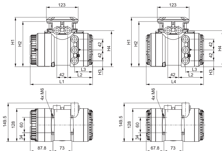
Рис. 21. Размеры измерительного преобразователя в мм (слева: измерительный преобразователь с дисплеем, справа: измерительный преобразователь без дисплея)
