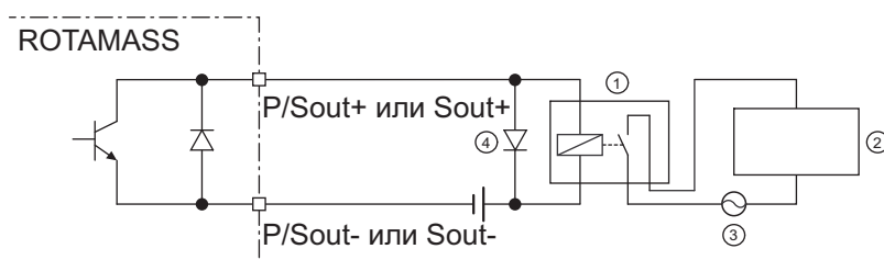
Рис. 34. Соединение пассивного выхода состояния P/Sout или Sout для цепи электромагнитного клапана
