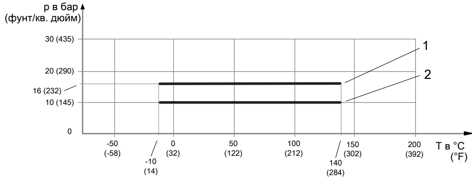
Рис. 14. Допустимое давление технологического процесса в зависимости от температуры в месте соединения с технологическим процессом
