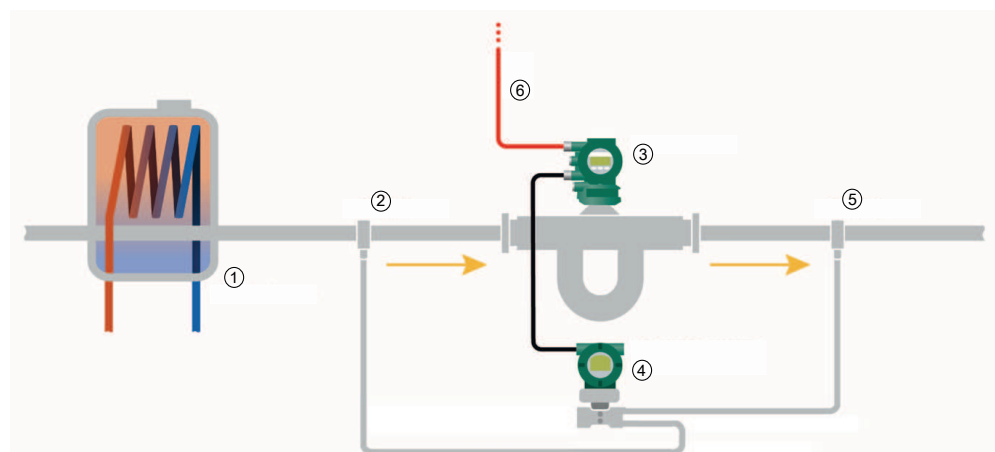
Рис. 41. Функция определения вязкости позволяет получить эталонное значение, используемое для активации системы нагрева (на приведенной выше диаграмме показаны основные функциональные возможности для одной или нескольких возможностей установки)
