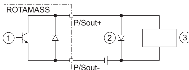
Рис. 30. Соединение пассивного импульсного выхода P/Sout с электромеханическим счетчиком
