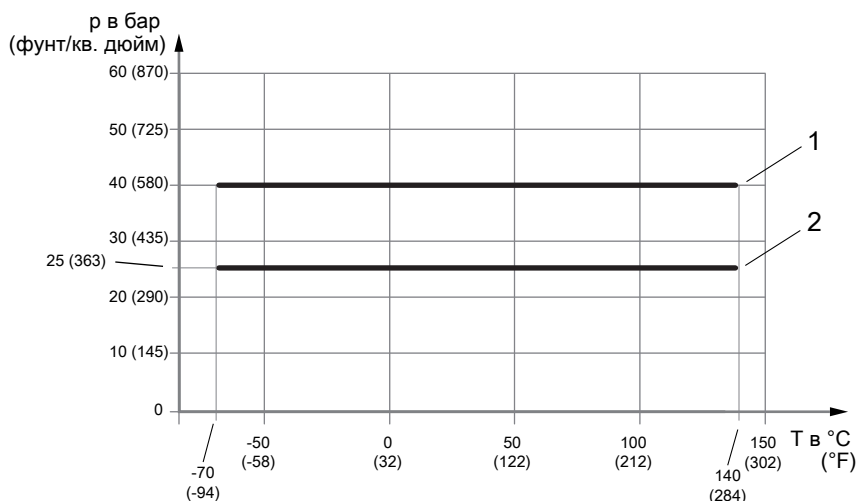
Рис. 12. Допустимое давление технологического процесса в зависимости от температуры в месте соединения с технологическим процессом
