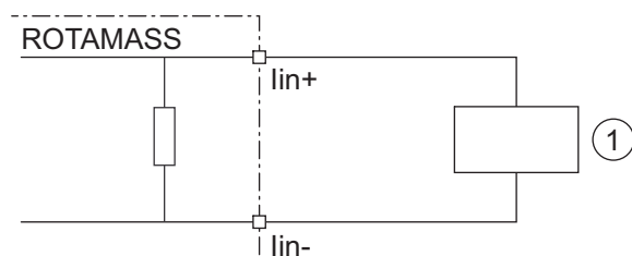
Рис. 37. Подсоединение внешнего устройства с активным токовым выходом
