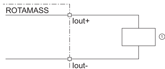
Рис. 23. Соединение активного токового выхода I out HART
