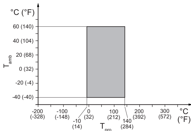
Рис. 16. Допустимая температура рабочей среды и окружающей среды, интегральное исполнение, для типа присоединения к технологическому процессу HS4 и HS8
