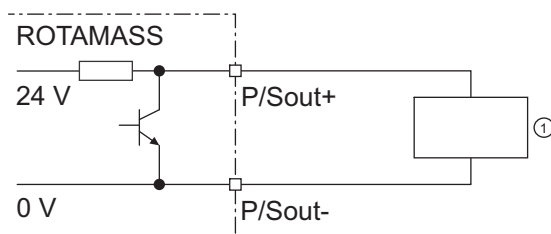
Рис. 28. Активный импульсный выход P/Sout с внутренним нагрузочным резистором
