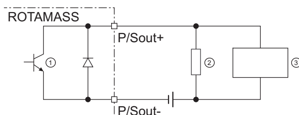
Рис. 29. Соединение пассивного импульсного выхода P/Sout с электронным счетчиком
