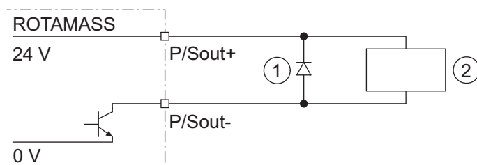
Рис. 27. Соединение активного импульсного выхода P/Sout с электромеханическим счетчиком
