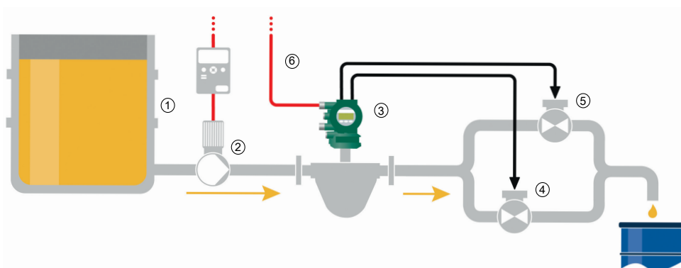
Рис. 40. Двухэтапный режим (на приведенной выше диаграмме показаны основные функциональные возможности для одной или нескольких возможностей комбинирования)
