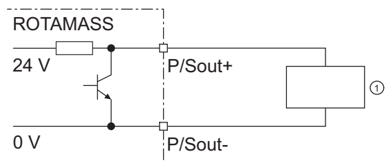
Рис. 32. Активный выход состояния P/Sout с внутренним нагрузочным резистором
