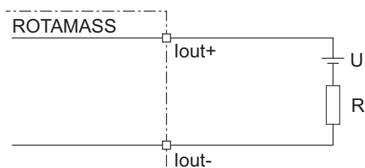
Рис. 25. Соединение пассивного токового выхода I out
