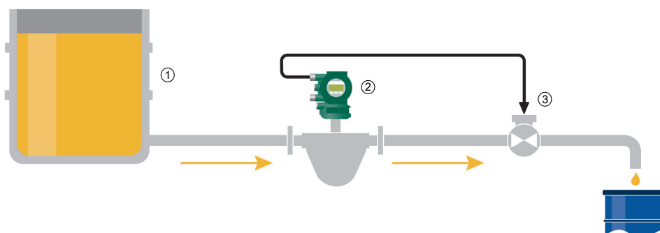
Рис. 39. Одноэтапный режим (на приведенной выше диаграмме показаны основные функциональные возможности для одной или нескольких возможностей комбинирования)
