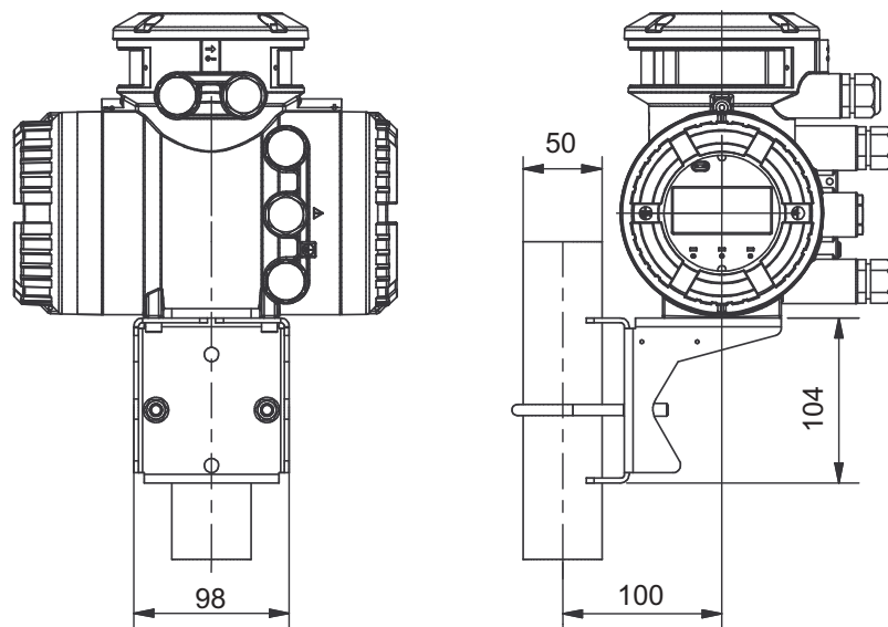
Рис. 22. Размеры измерительного преобразователя в мм, присоединен при помощи консоли из листовой стали (кронштейн)
