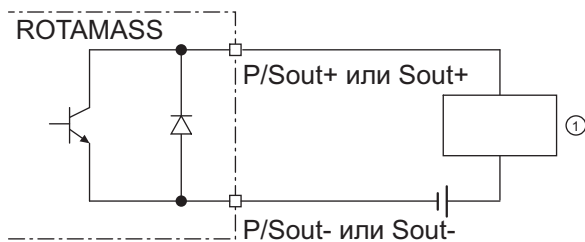
Рис. 33. Соединение пассивного выхода состояния P/Sout или Sout
