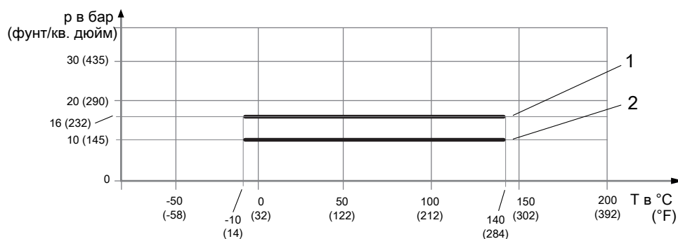
Рис. 13. Допустимое давление технологического процесса в зависимости от температуры в месте соединения с технологическим процессом
