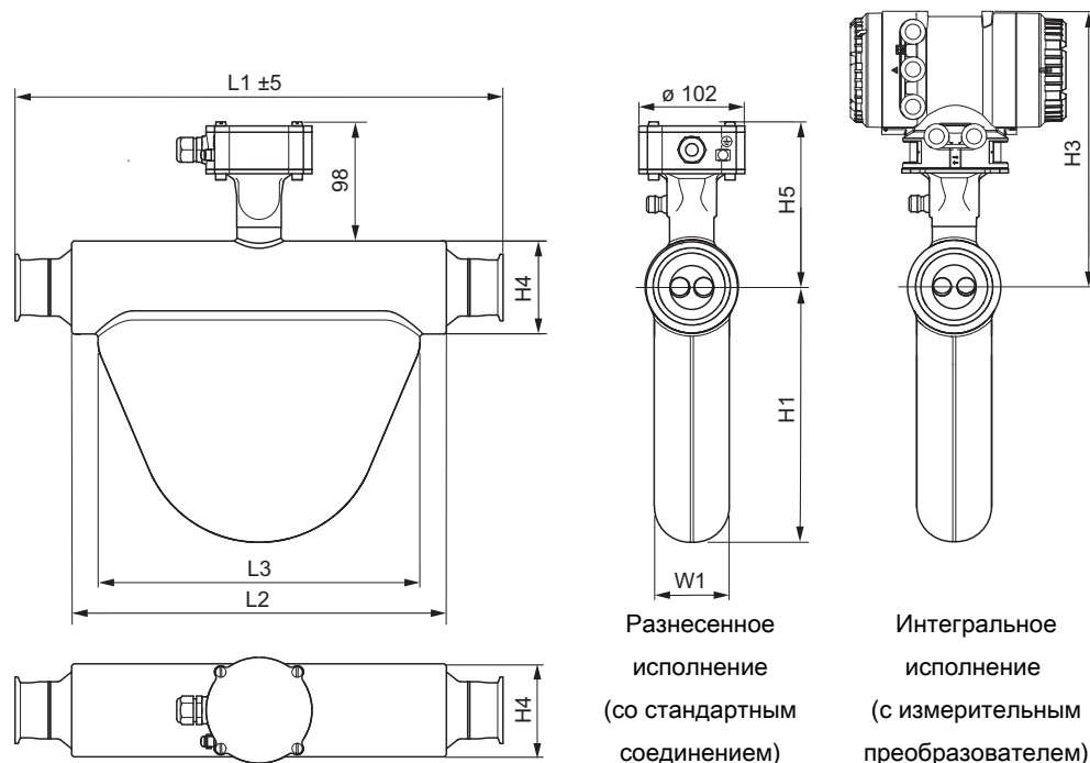
Рис. 20. Размеры в мм
