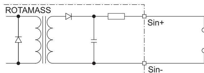
Рис. 38. Соединение входа состояния
