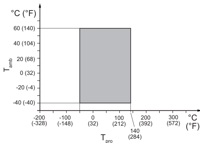
Рис. 15. Допустимая температура рабочей среды и окружающей среды, интегральное исполнение, для типа присоединения к технологическому процессу HS2
