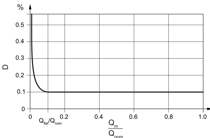
Рис. 9. Схема зависимости максимального отклонения от массового расхода
