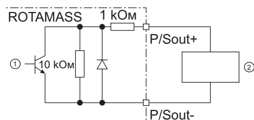
Рис. 35. Пассивный выход или выход состояния с соединенным последовательно коммутирующим усилителем
