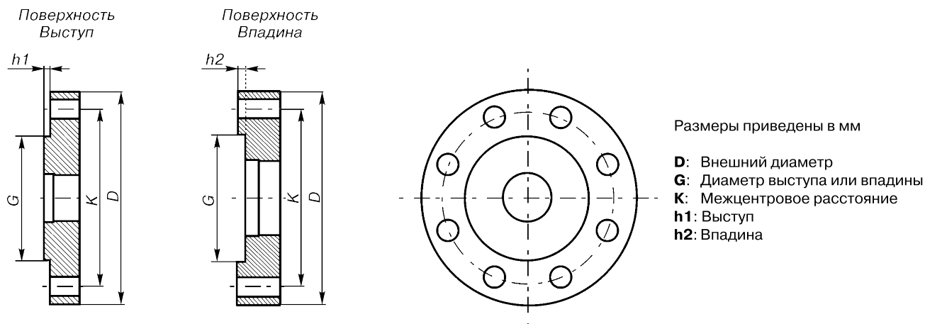
Рис. 12. Размеры фланцев.
