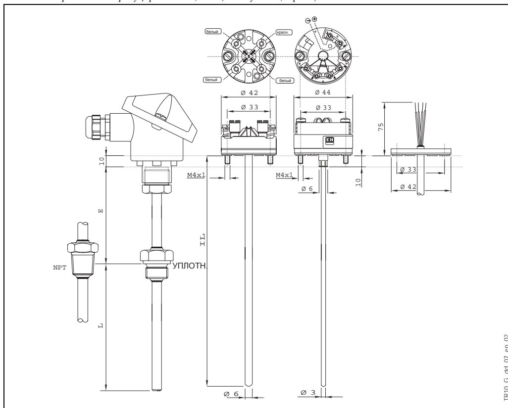
Рис. 11: Рабочие компоненты
