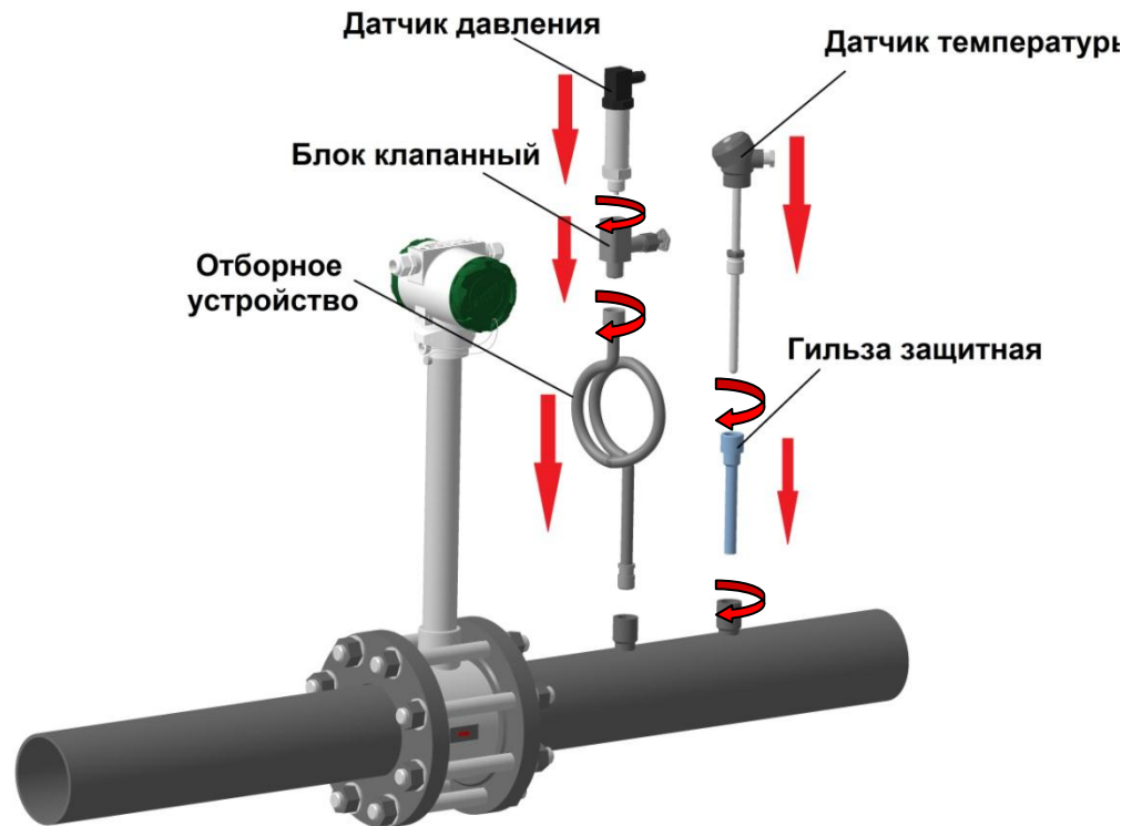
Рисунок 2.4 – Схема монтажа преобразователя давления и преобразователя температуры
