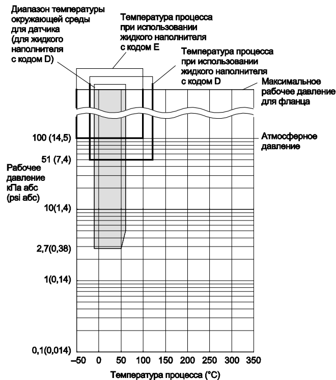
Рисунок 1-2. Рабочее давление и температура процесса (Жидкий наполнитель: фторированное масло для использования при недопустимости присутствия масел и этиленгликоль для низкотемпературного применения)
